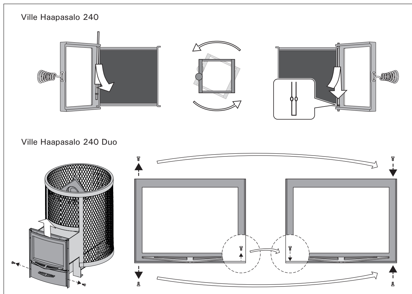
Рисунок 13. Изменение стороны подвески дверцы каменки
