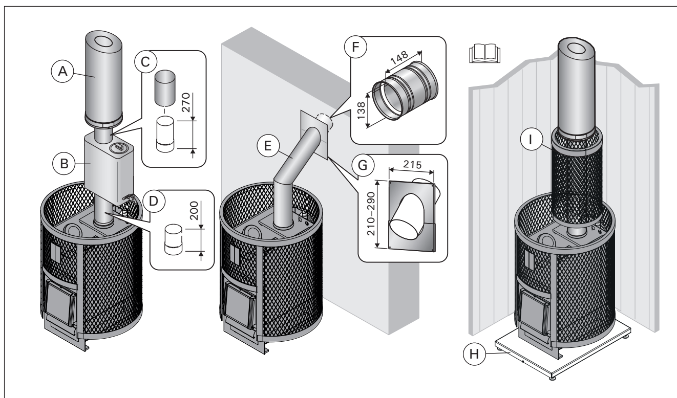
Рисунок 15. Дополнительные принадлежности (все размеры приведены в миллиметрах)
