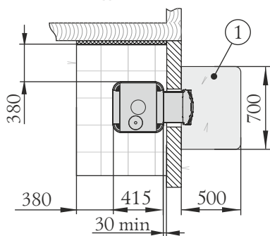
Вид А
