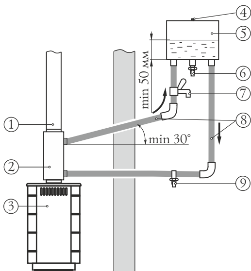
Рисунок 6. Схема монтажа системы водонагрева с использованием теплообменника «Костакан».
